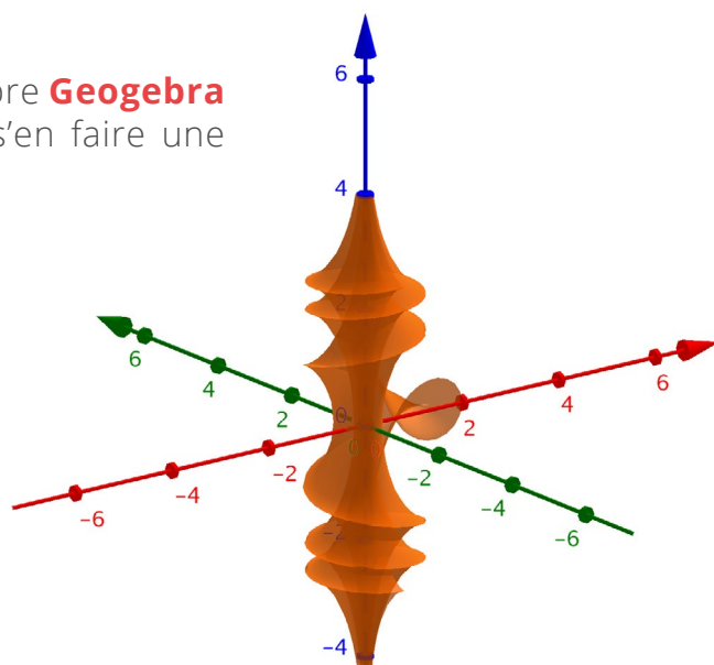
Représentation de la surface de Kuen pour u entre 0 et 6\pi et v entre -6 et 6.
